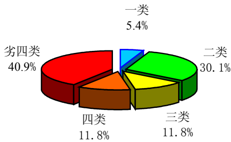
东海海区水质状况
