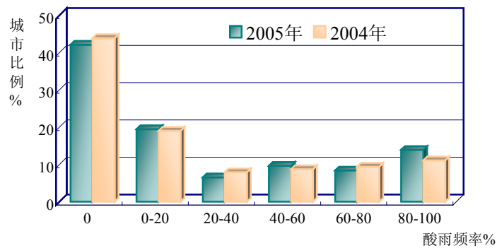
不同酸雨频率城市比例
