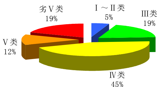
2005年松花江水系水质类别比例分布
