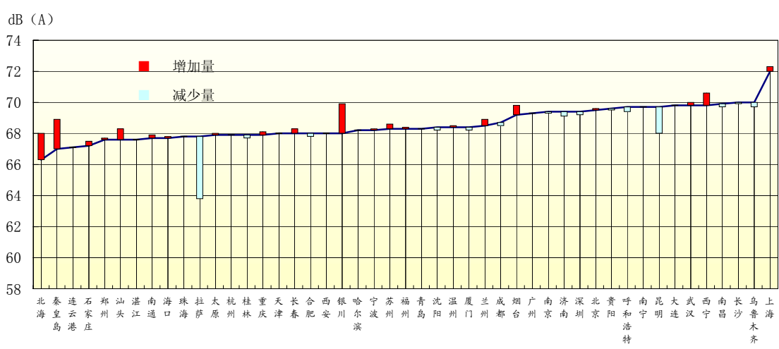
2005 年 47 个重点城市道路交通噪声等效声级年际比较
