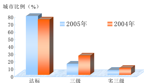
二氧化硫浓度分级城市比例
