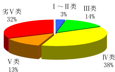
2005年淮河水系水质类别比例分布
