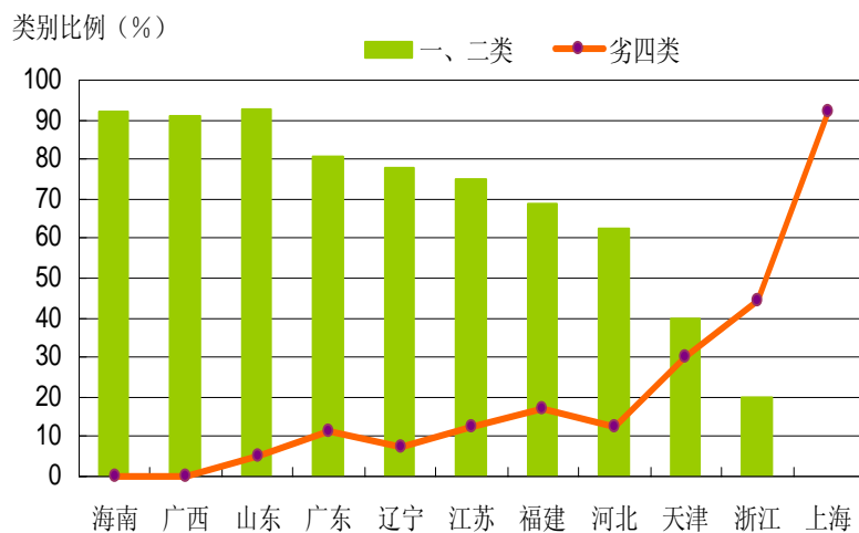
2005 年沿海省、自治区、直辖市近岸海域海水水质类别
