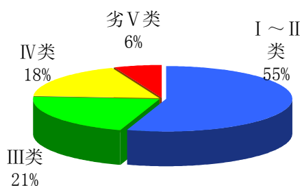
2005年珠江水系水质类别比例分布
